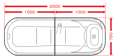
浴槽寸法図【単位:mm】
