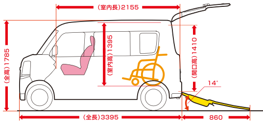
車両寸法図・室内レイアウト[単位:mm]
