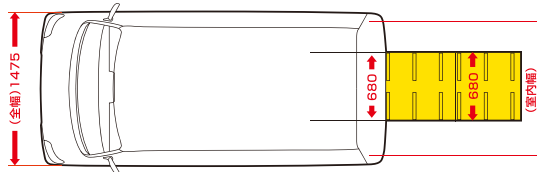
リヤシート付仕様車(5ナンバー) 室内レイアウト
