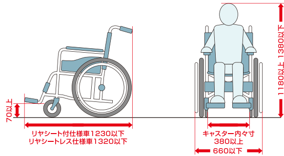
車いす乗車の目安[単位:mm]
