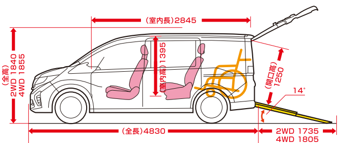
車両寸法図〔単位:mm〕
