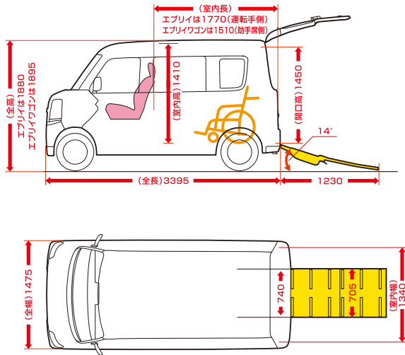
車両寸法図〔単位:mm〕
