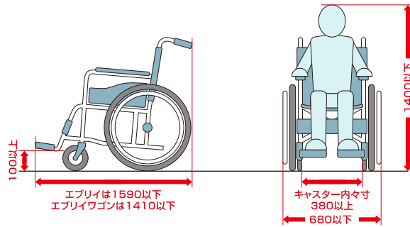
車いす乗車の目安〔単位:mm〕
