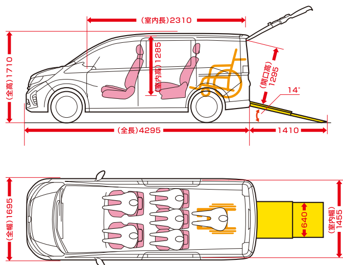
車両寸法図〔単位:mm〕
