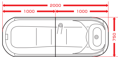
浴槽寸法図 [単位:mm]
